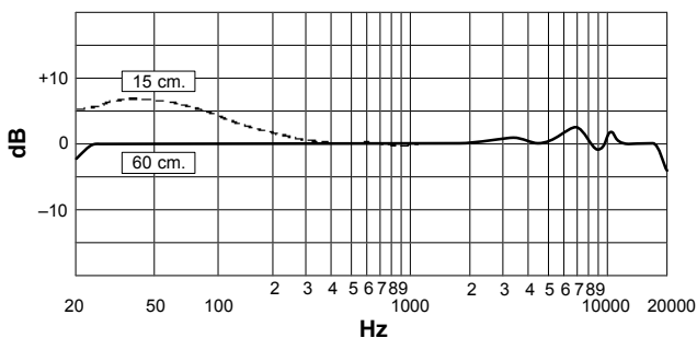
FIGURA 4. RESPUESTA DE FRECUENCIA TYPICA
