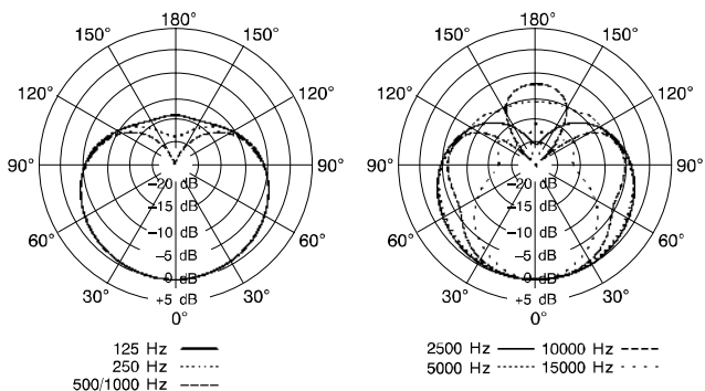
FIGURA 5. PATRONES DE CAPTACION POLAR TYPICOS
